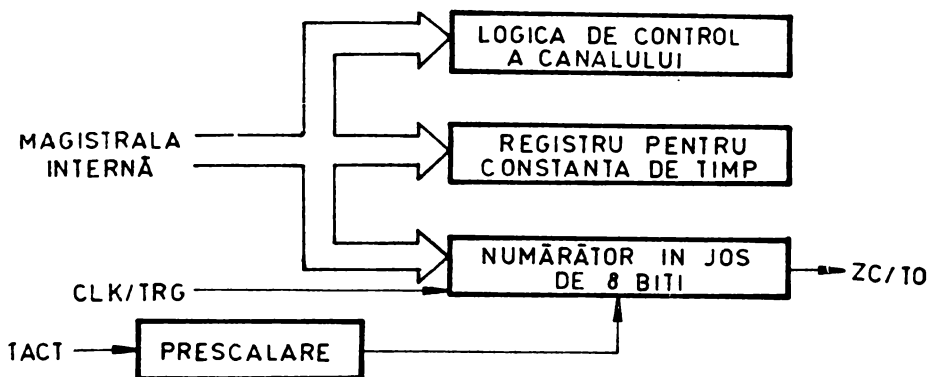
Fig. 4.2 Diagrama bloc a unui numărător/temporizator.
