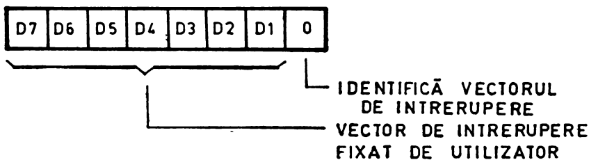
Fig. 6.5 Cuvîntul vector de întrerupere.
