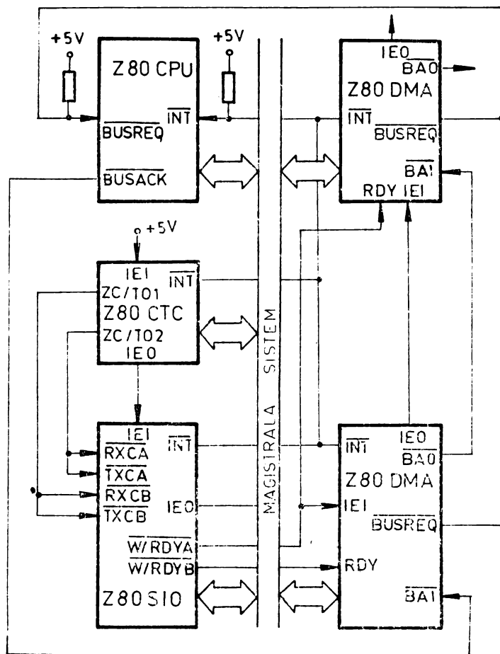
Fig. 7.3 Sistem Z80 tipic.
