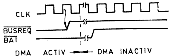
Fig. 7.15 Eliberarea magistralei (modul „cite un octet”).
