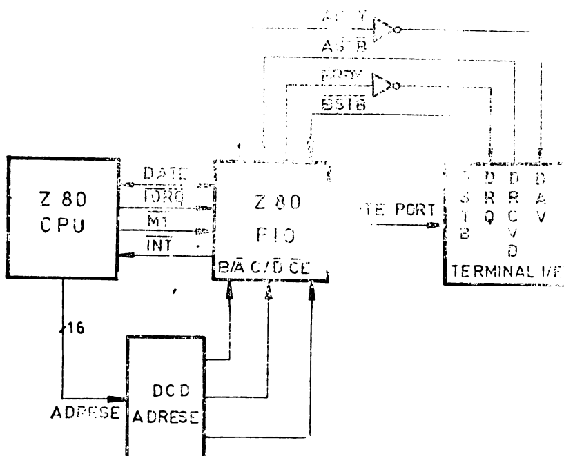
Fig. 6.18 Exemplu de interfață de intrare/ieșire.
