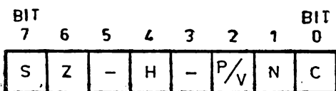
Fig. 3.10 Registrul indicatorilor de condiții.
