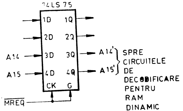
Fig. 8.24 Captarea biților superiori de adresă.
