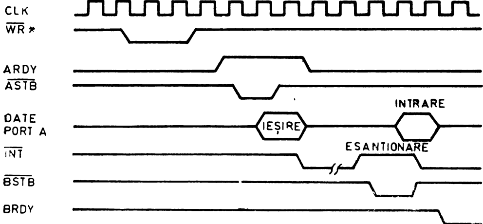
Fig. 6.13 Diagramă în timp pentru modul 2.
