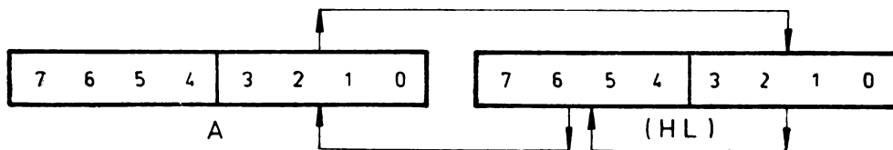
Fig. 3.6 Efectul instrucțiunii RRD.
