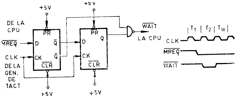
Fig. 8.15 Adăugarea unei stări de așteptare la fiecare ciclu de acces la memorie.
