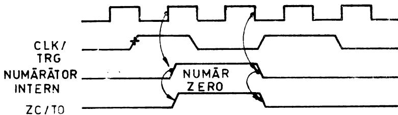
Fig. 4.9 Diagramă în timp pentru modul de numărător.
