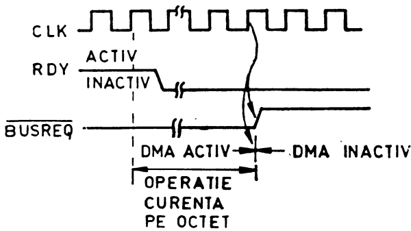
Fig. 7.17 Eliberarea magistralei la semnal RDY inactiv.
