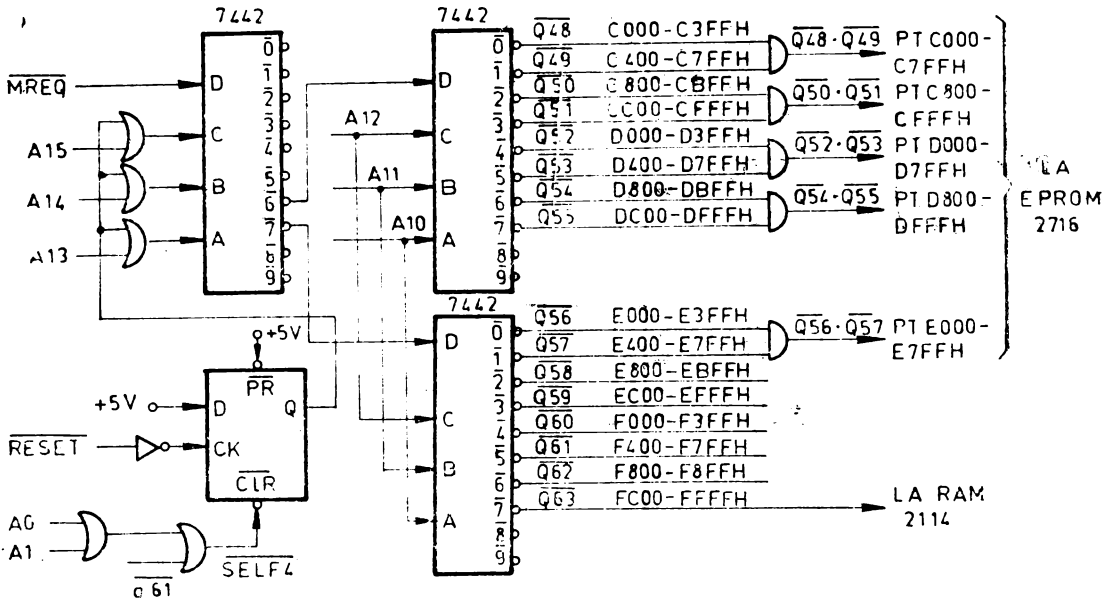
Fig. 8.11 Generarea semnalelor de selecție a memoriilor, pentru spații de 1 ko.
