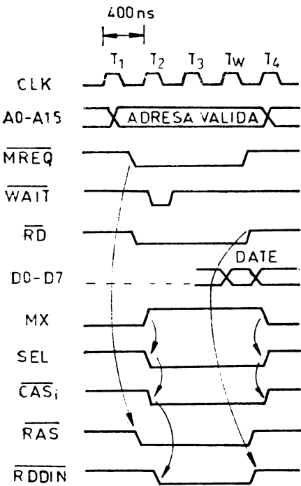
Fig. 8.23 Citirea memoriilor RAM dinamic.
