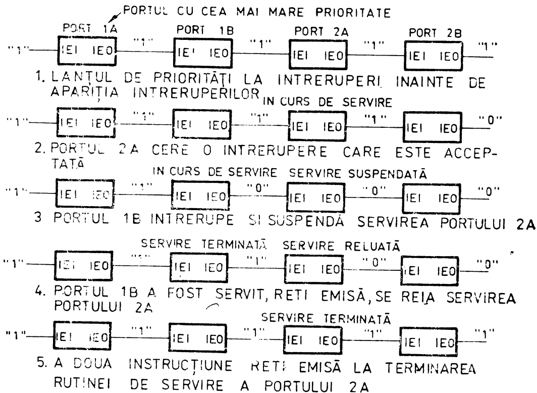
Fig. 6.16 Servirea întreruperilor într-un lanț de priorități.
