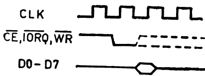
Fig. 7.9 Ciclu de scriere CPU → DMA.
