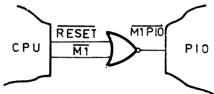
Fig. 6.3 Inițializarea circuitului Z80 PIO.
