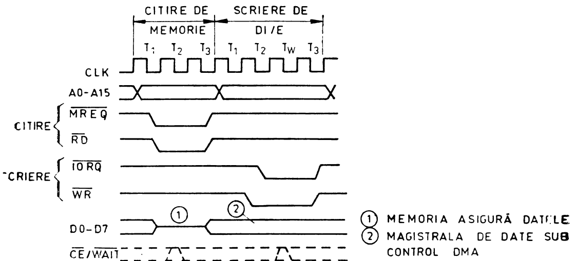
Fig. 7.11 Transfer de la memorie spre DI/E.
