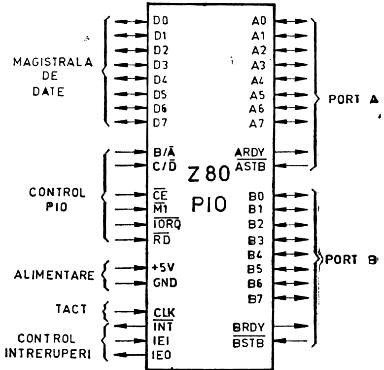
Fig. 6.10 Funcțiile logice ale circuitului Z80 PIO.
