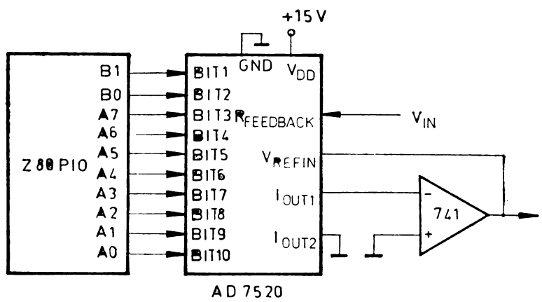
Fig. 8.29 Divizarea analog/numerică realizată cu circuitul AD7520.
