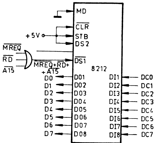
Fig. 8.19 Condiționarea deschiderii căii de citire a datelor dintr-o zonă a memoriei (se deschide pentru jumătatea superioară).
