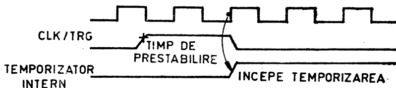
Fig. 4.8 Diagramă în timp pentru modul de temporizator.
