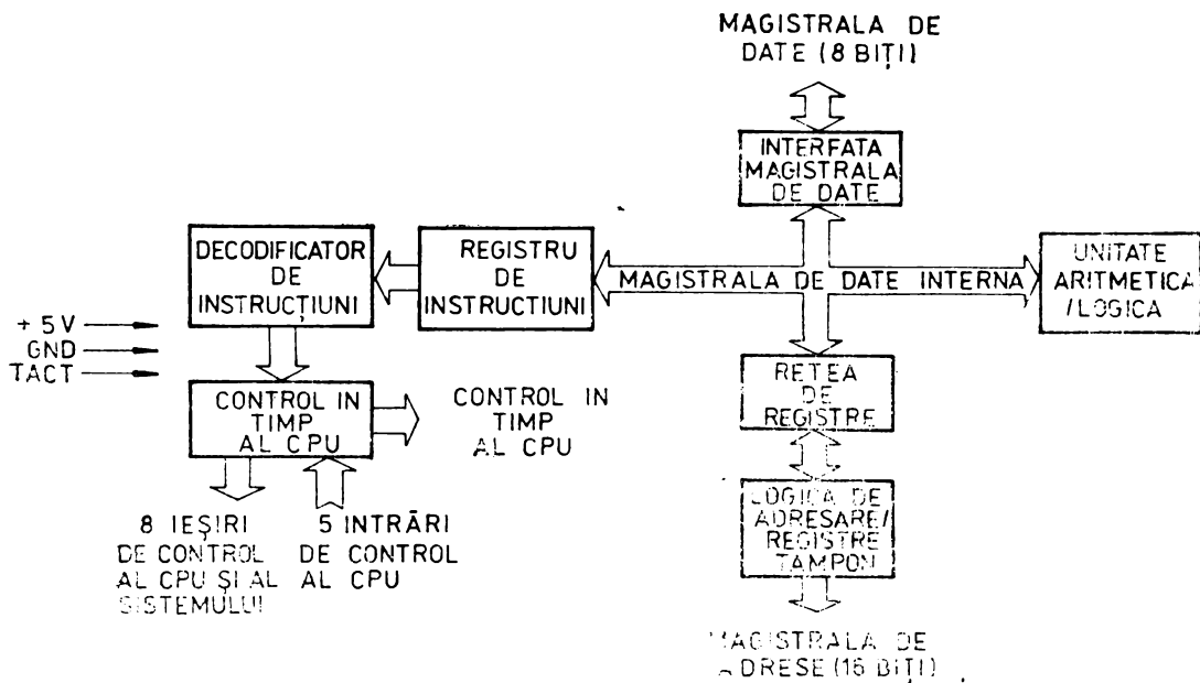
Fig. 2.1 Schema bloc a unității centrale Z80 CPU.
