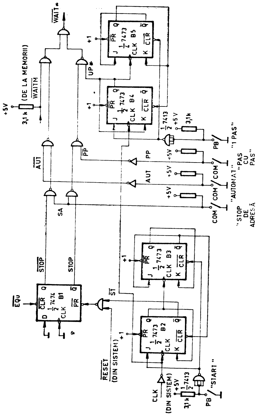
Fig. 8.32 Circuitul de generare a semnalului de așteptare, \overline{\text{WAIT}}^* .
