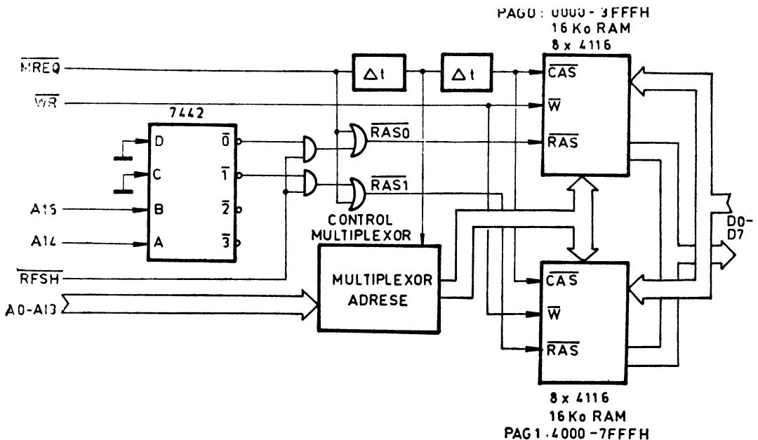
Fig. 8.21 Interfașarea memoriilor RAM dinamic 4116 ( \overline{\text{CAS}} comun).
