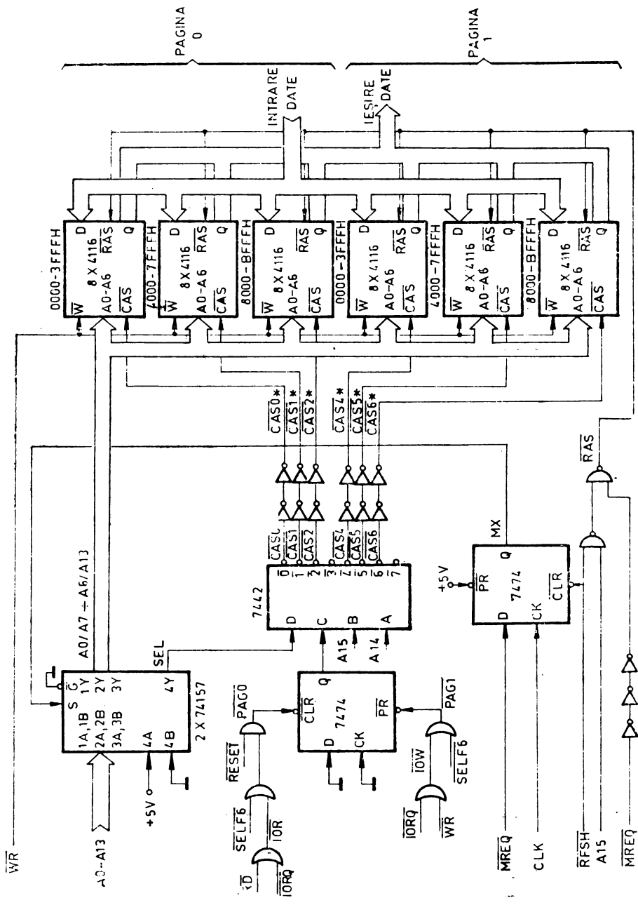
Fig. 8.26 Extinderea capacității memoriei sistemului peste 64 ko.
