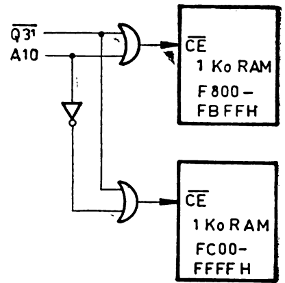
Fig. 8.10 Complectarea decodificării cu porți.
