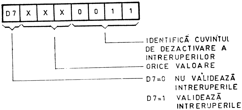
Fig. 6.9 Cuvîntul de dezactivare a intreruperilor.
