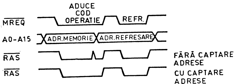
Fig. 8.25 Semnalul \overline{\text{RAS}} cu și fără captarea adreselor.
