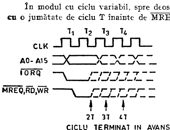
Fig. 7.13 Desfășurarea în timp a ciclurilor variabile și a fronturilor.
