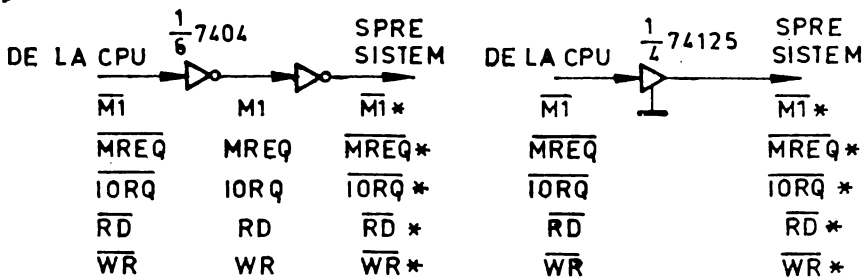
Fig. 8.16 Amplificarea/separarea unor semnale de control emise de unitatea centrală.
