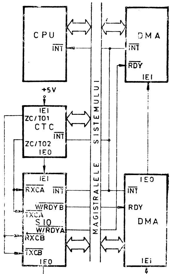
Fig. 5.6 Sistem Z80 tipic.
