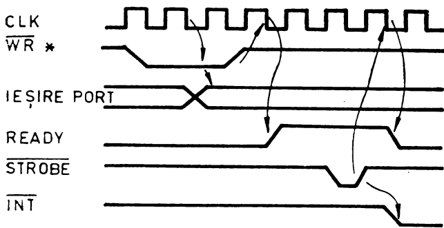
Fig. 6.11 Diagramă în timp pentru modul 0.
