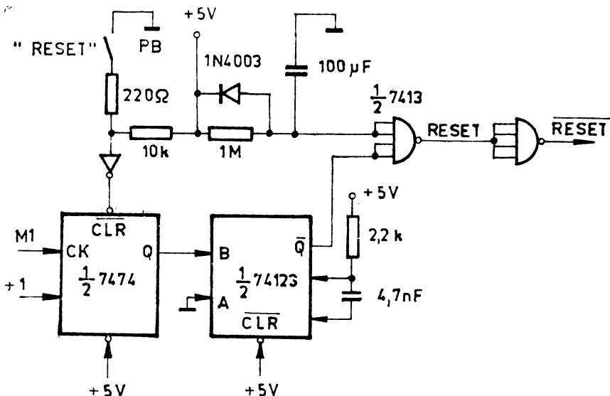
Fig. 8.5 Logică de inițializare.
