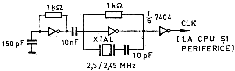
Fig. 8.2 Oscilator cu cristal de cuarț de 2,5 MHz.
