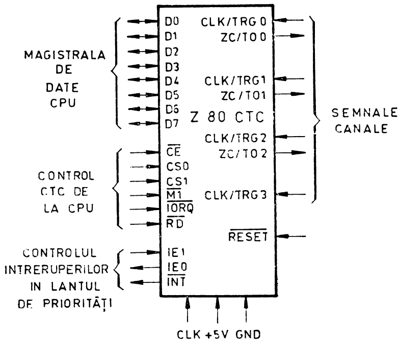
Fig. 4.6 Funcțiile logice ale circuitului Z80 CTC.
