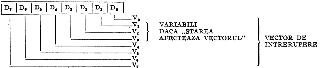
Fig. 5.7 Funcțiile biților din registrele de citire.
