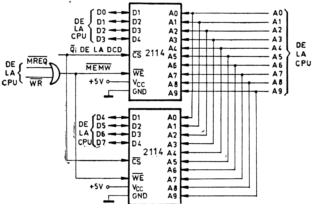
Fig. 8.13 Conectarea memoriilor RAM 2114.
