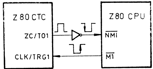
Fig. 4.13 Conexiuni Z80 CTC—Z80 CPU pentru rulara pas cu pas a unui program.
