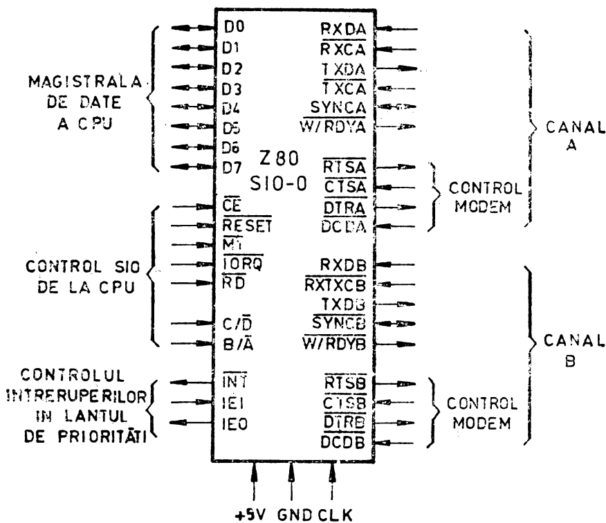
Fig. 5.1 Funcțiile logice ale circuitului Z80 SIO-0.
