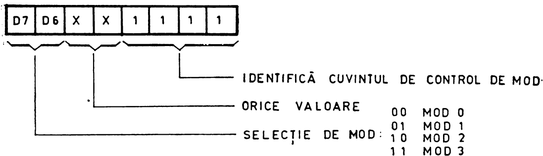
Fig. 6.4 Cuvintul de control de mod.
