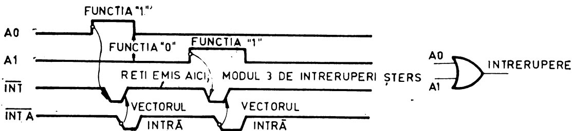
Fig. 6.15 Exemflu de întrerupere în modul 3.
