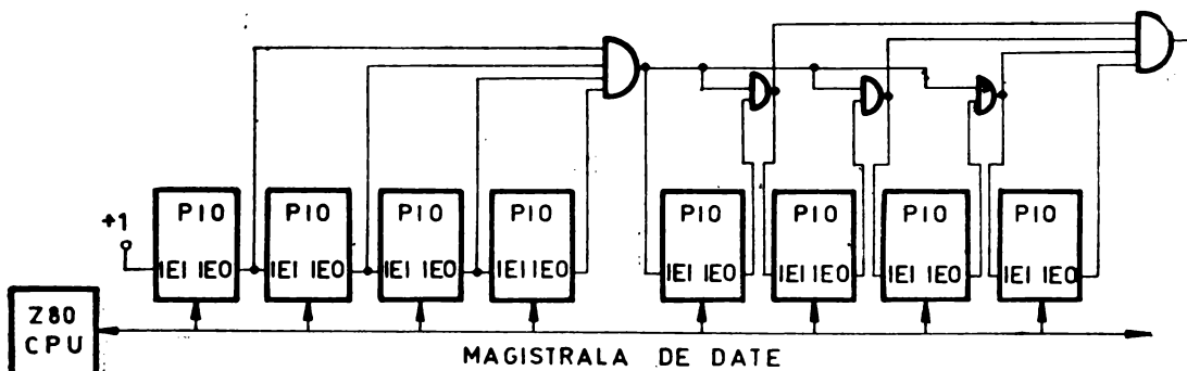
Fig. 6.17 Metode de extindere a lanțului de prioritați.
